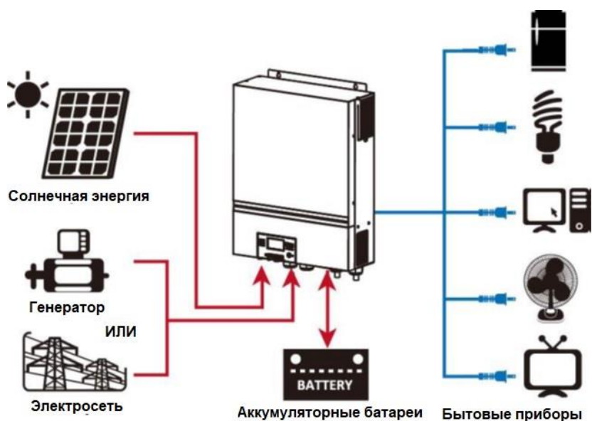
Рисунок 1. Общая структурная схема гибридной фотоэлектрической системы.
