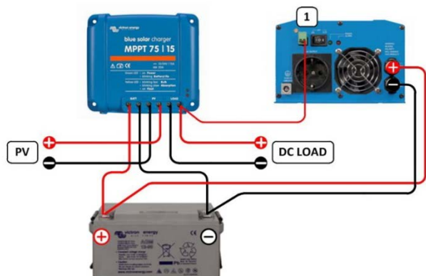
Рисунок 5: Инверторы Victron моделей Phoenix 12/800, 24/800, 12/1200 и 24/1200 можно контролировать, подключив правую сторону (1) удаленного пульта напрямую к выходу для нагрузок. Таким же образом, все инверторы Phoenix VE.Direct также можно контролировать, подключив левую сторону удаленного пульта к выходу для нагрузок.
